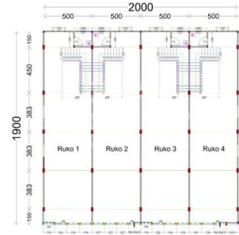
DENAH BANGUNAN LANTAI 2
