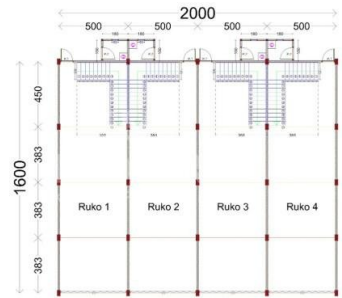
DENAH BANGUNAN LANTAI 1
